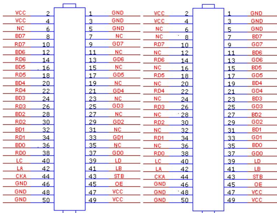
通用全彩接口一
